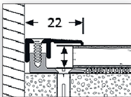
Abschlussprofil
