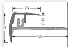
Treppenprofil
