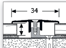
Übergangprofil
